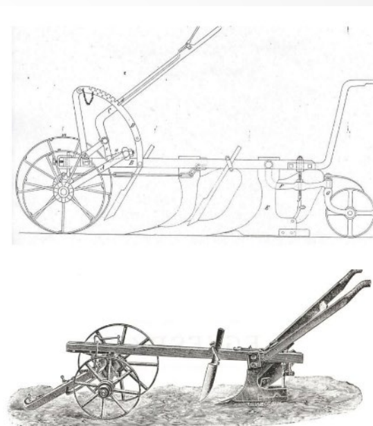
Patent János Lábassy Ungarn
